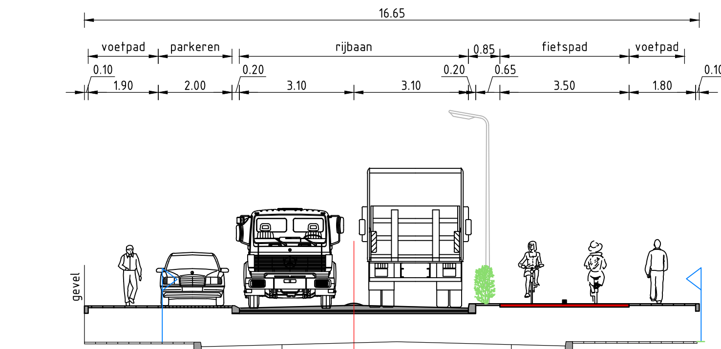
Dwarsprofiel 2 SCHAAL 1:100
