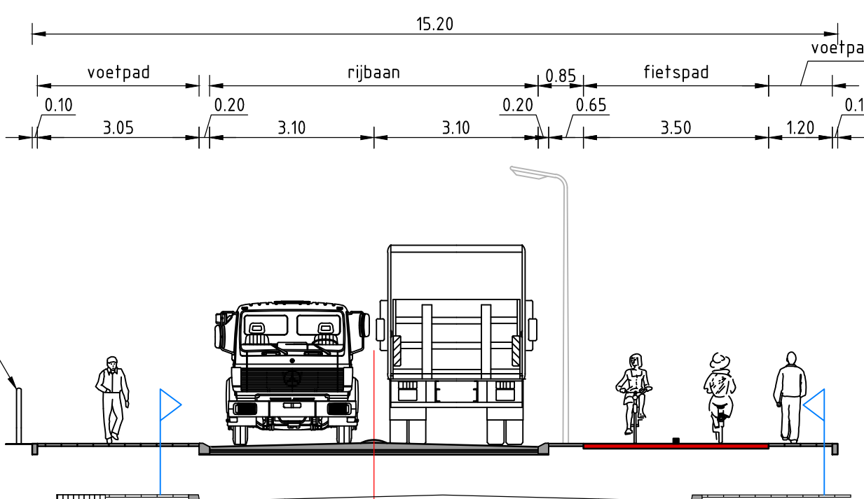
Dwarsprofiel 4 SCHAAL 1:100
