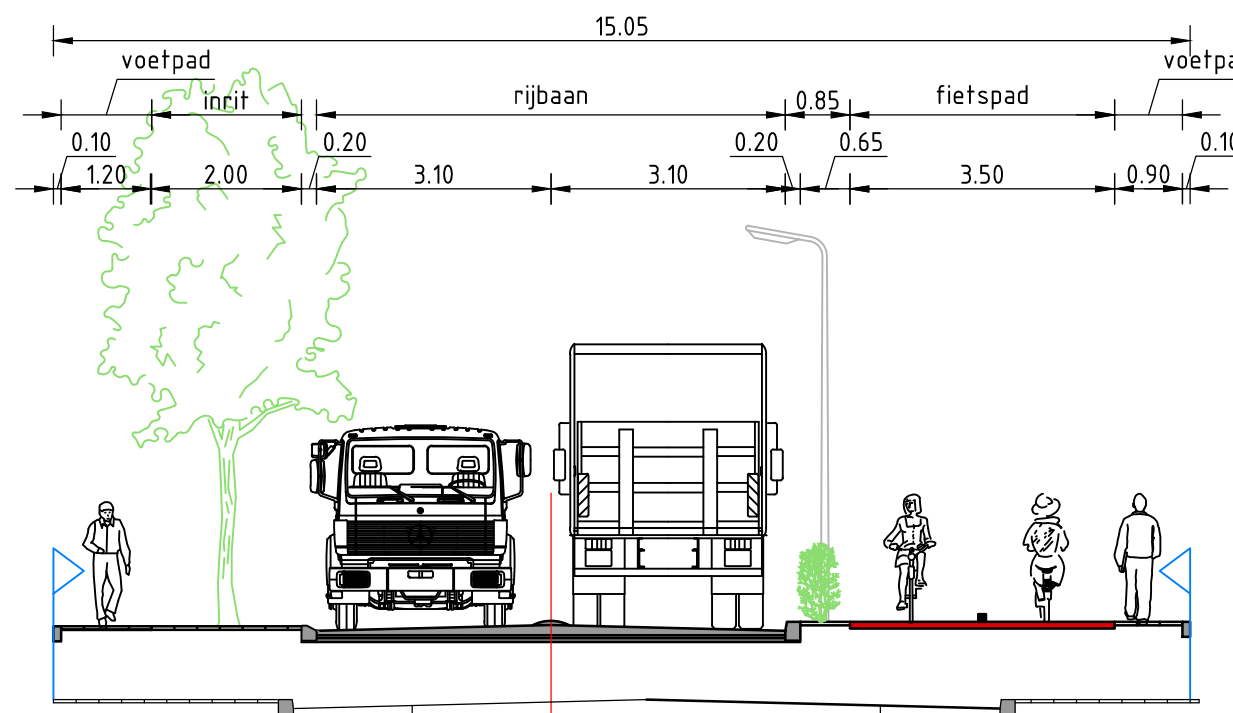
Dwarsprofiel 3 SCHAAL 1:100
