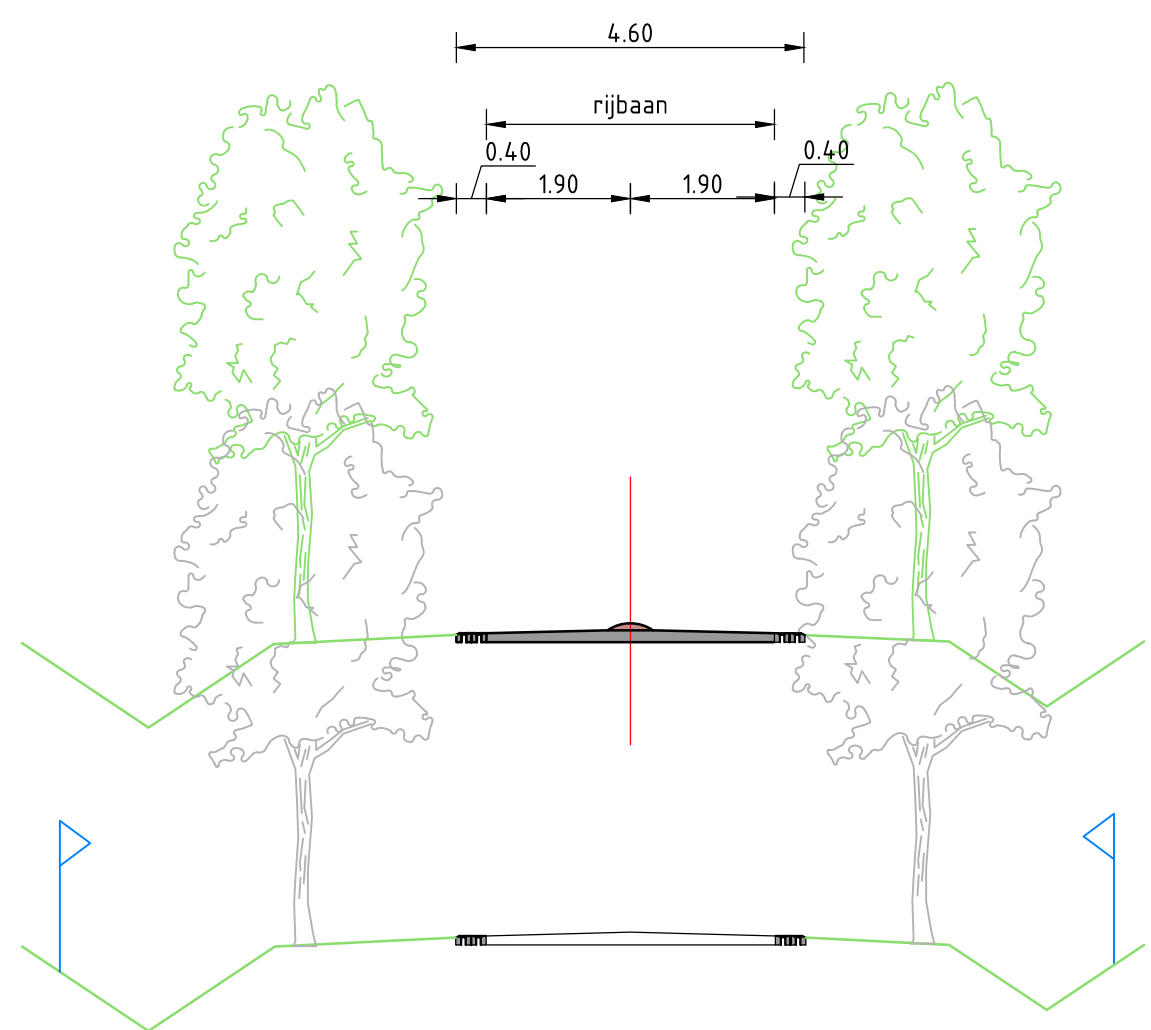
Dwarsprofiel 1 SCHAAAL 1:100
