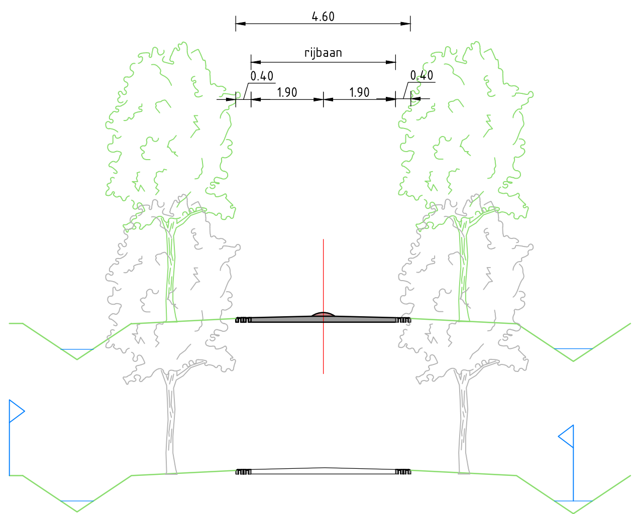
Dwarsprofiel 2
