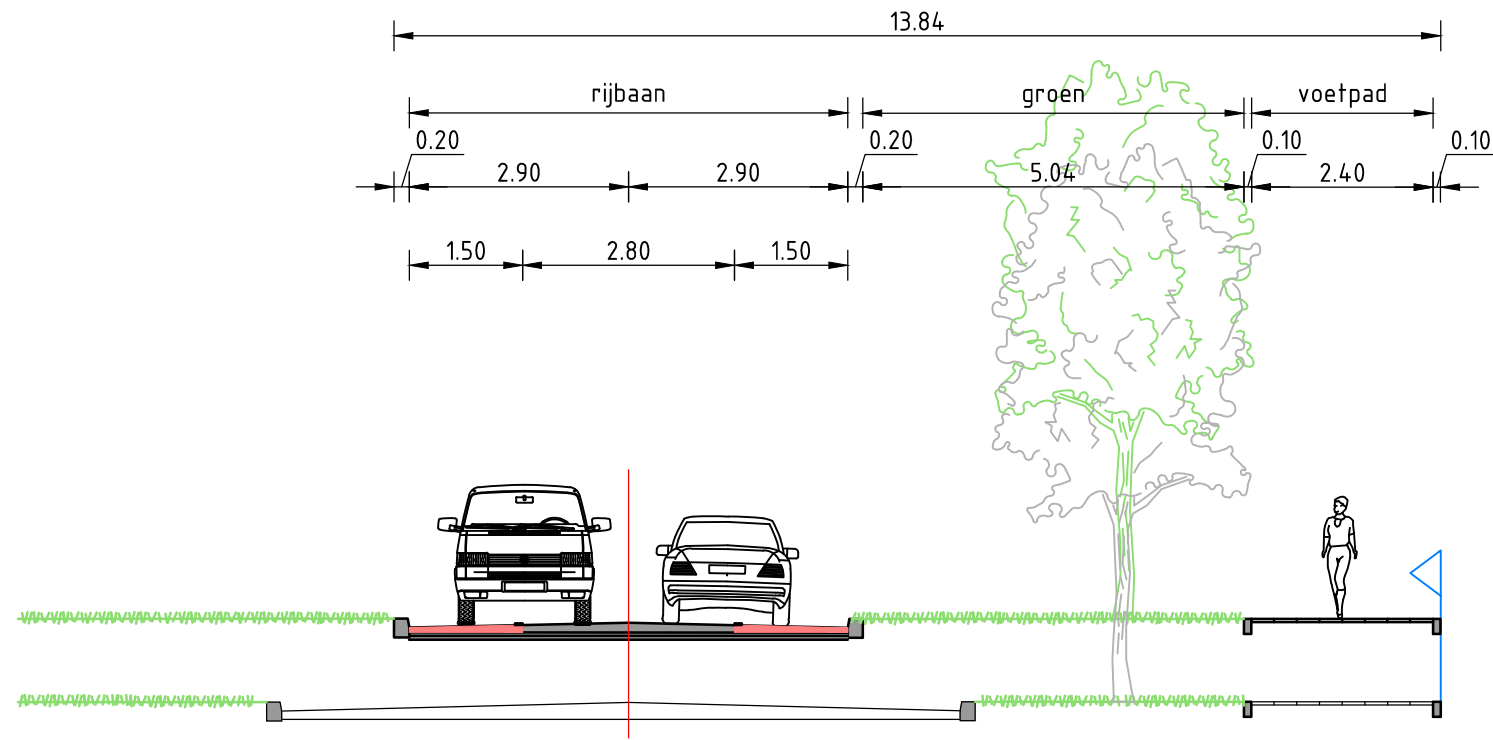
Dwarsprofiel 3 SCHAAL 1:100
