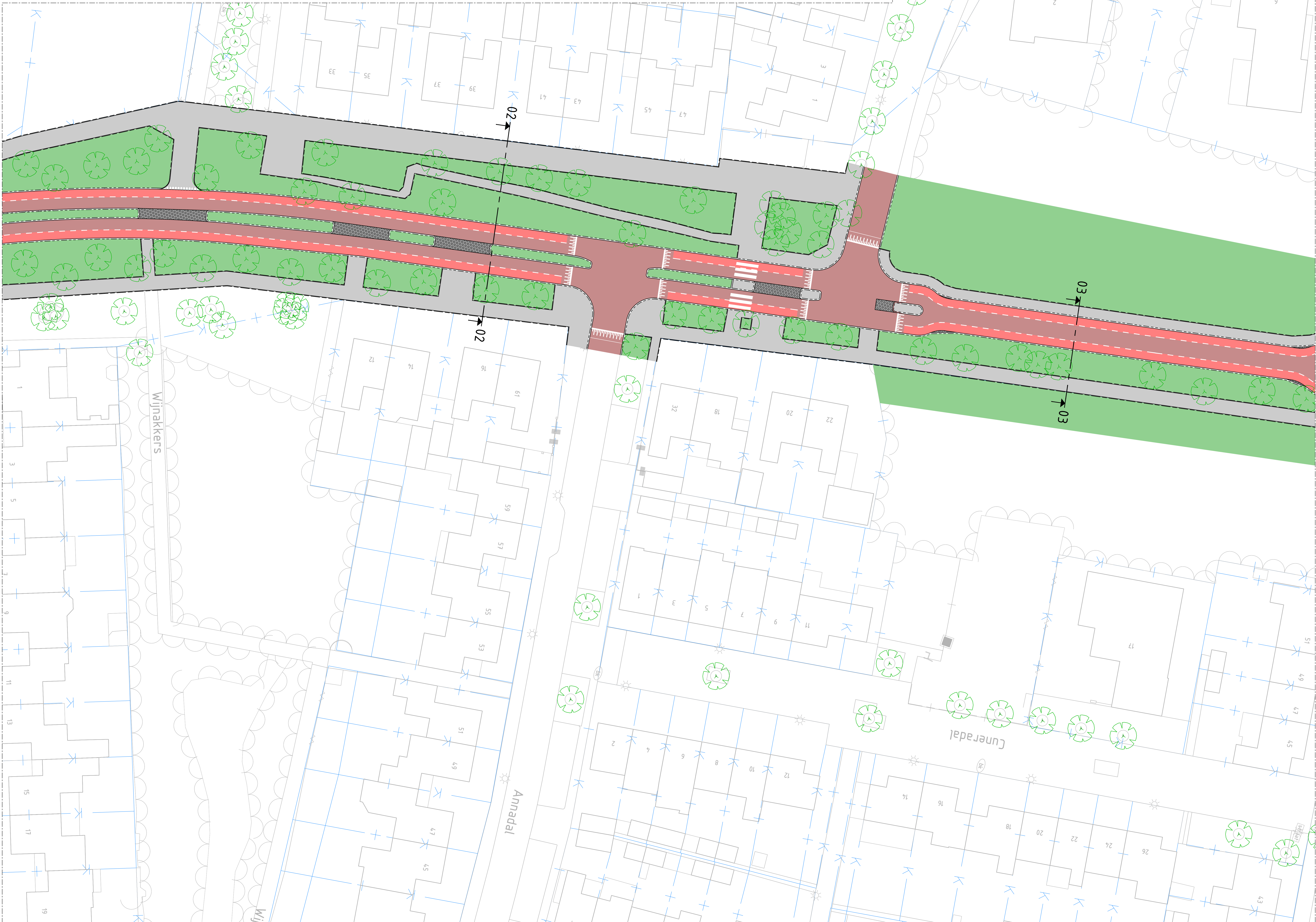
SITUATIETEKENING SCHAAL 1:250
