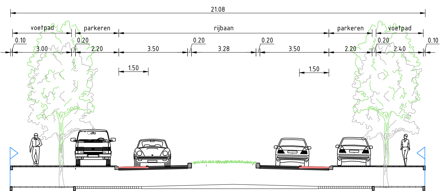
Dwarsprofiel 4 SCHAAL 1:100
