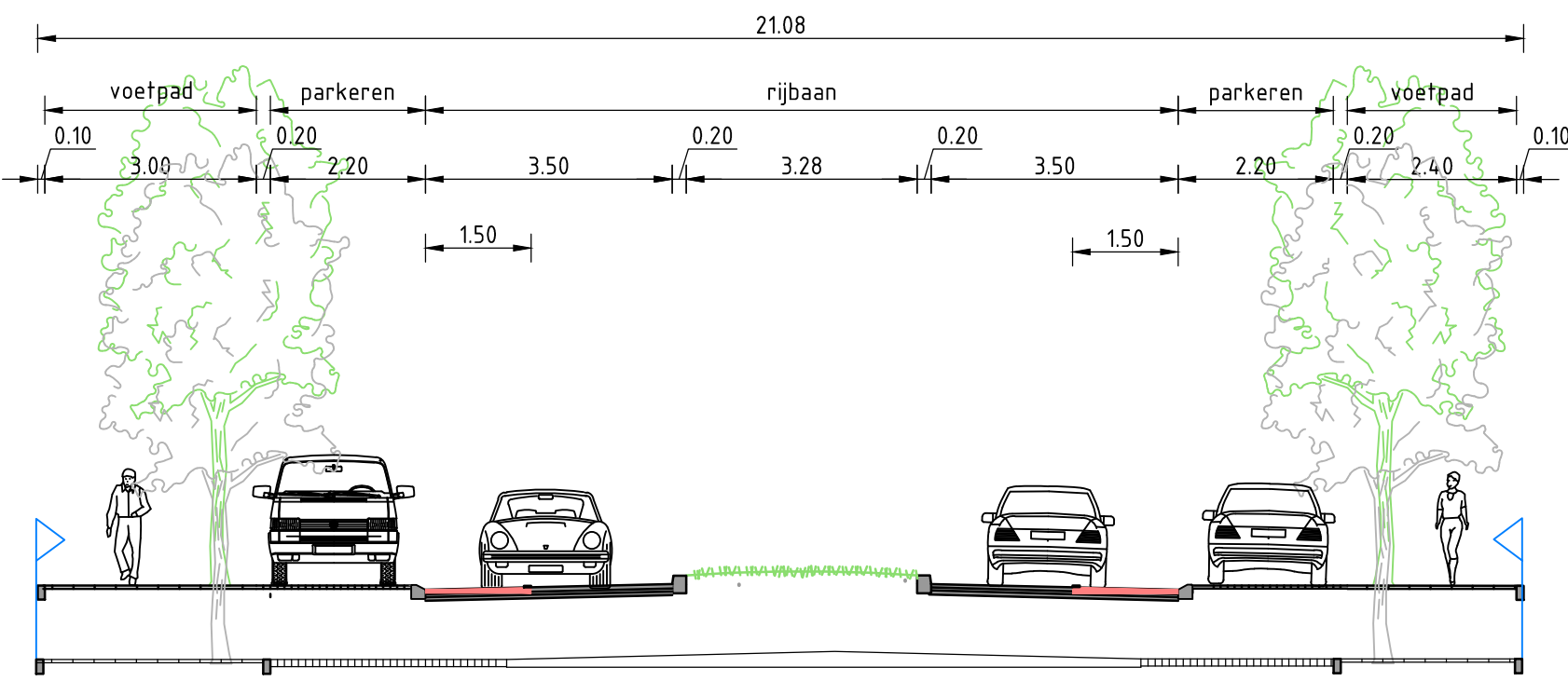
Dwarsprofiel 4 SCHAAL 1:100
