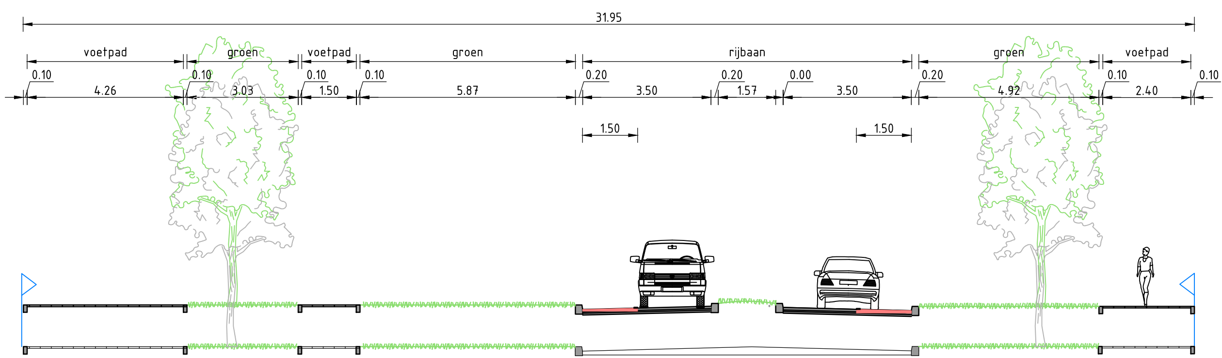
Dwarsprofiel 2 SCHAAL 1:100
