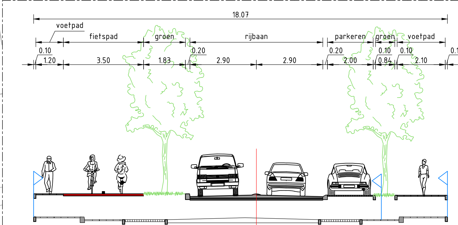
Dwarsprofiel 2 SCHAALE 1:100
