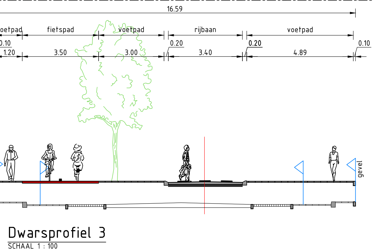
Dwarsprofiel 3 SCHAAL 1:100
