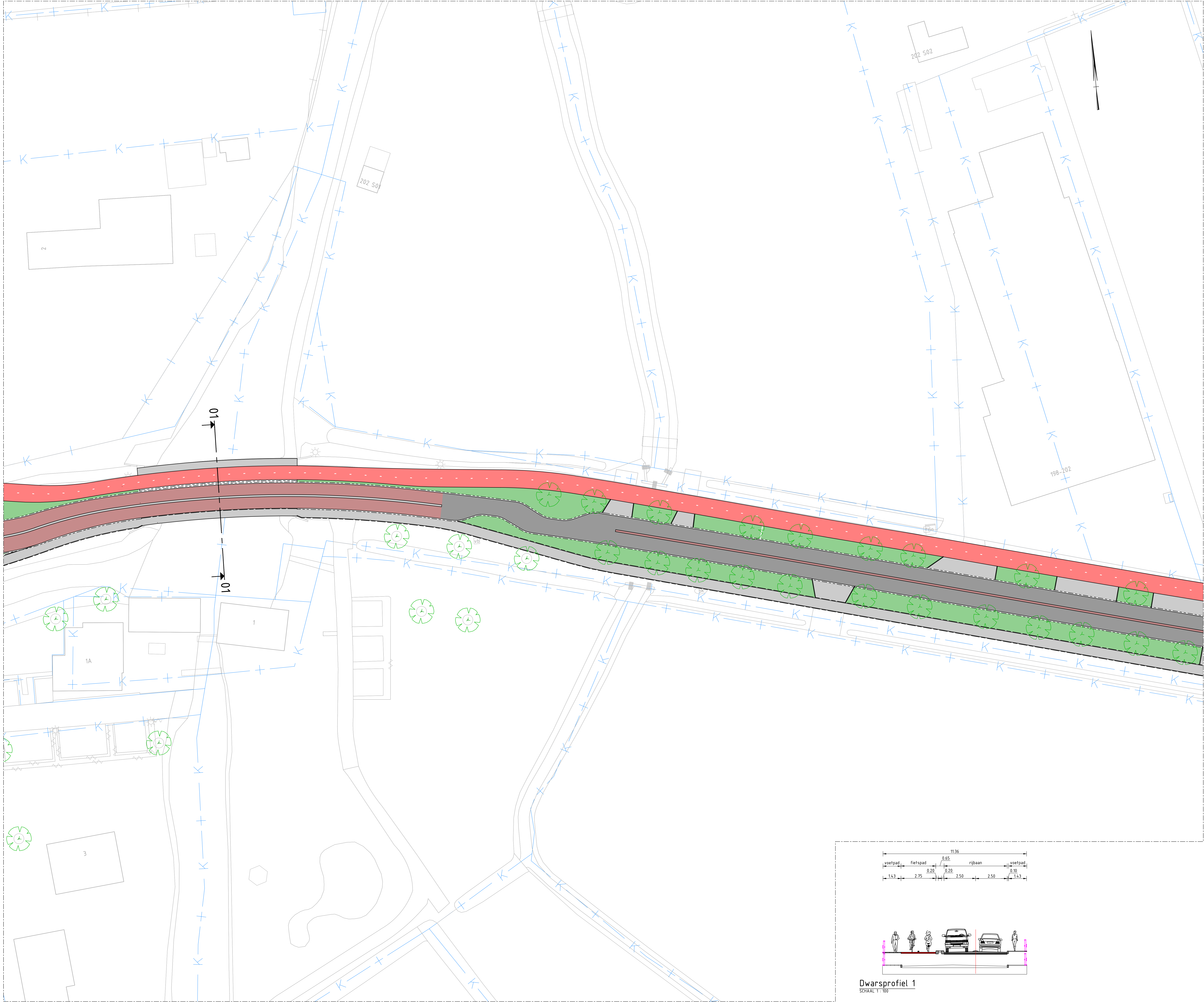
SITUATIETEKENING SCHAALE 1:250
