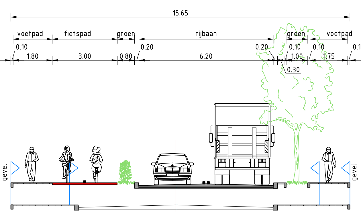
Dwarsprofiel 5 SCHAALE 1:100
