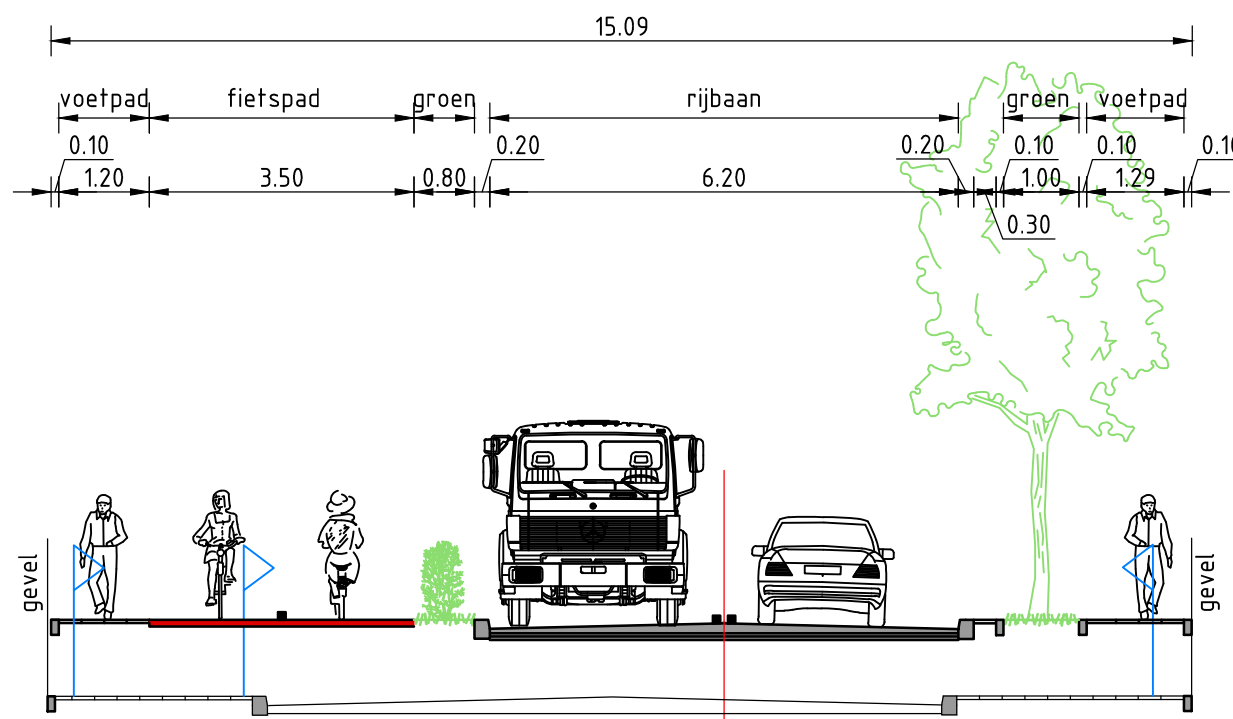
Dwarsprofiel 4 SCHAALE 1:100
