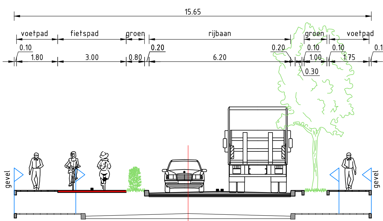
Dwarsprofiel 5 SCHAAL 1:100
