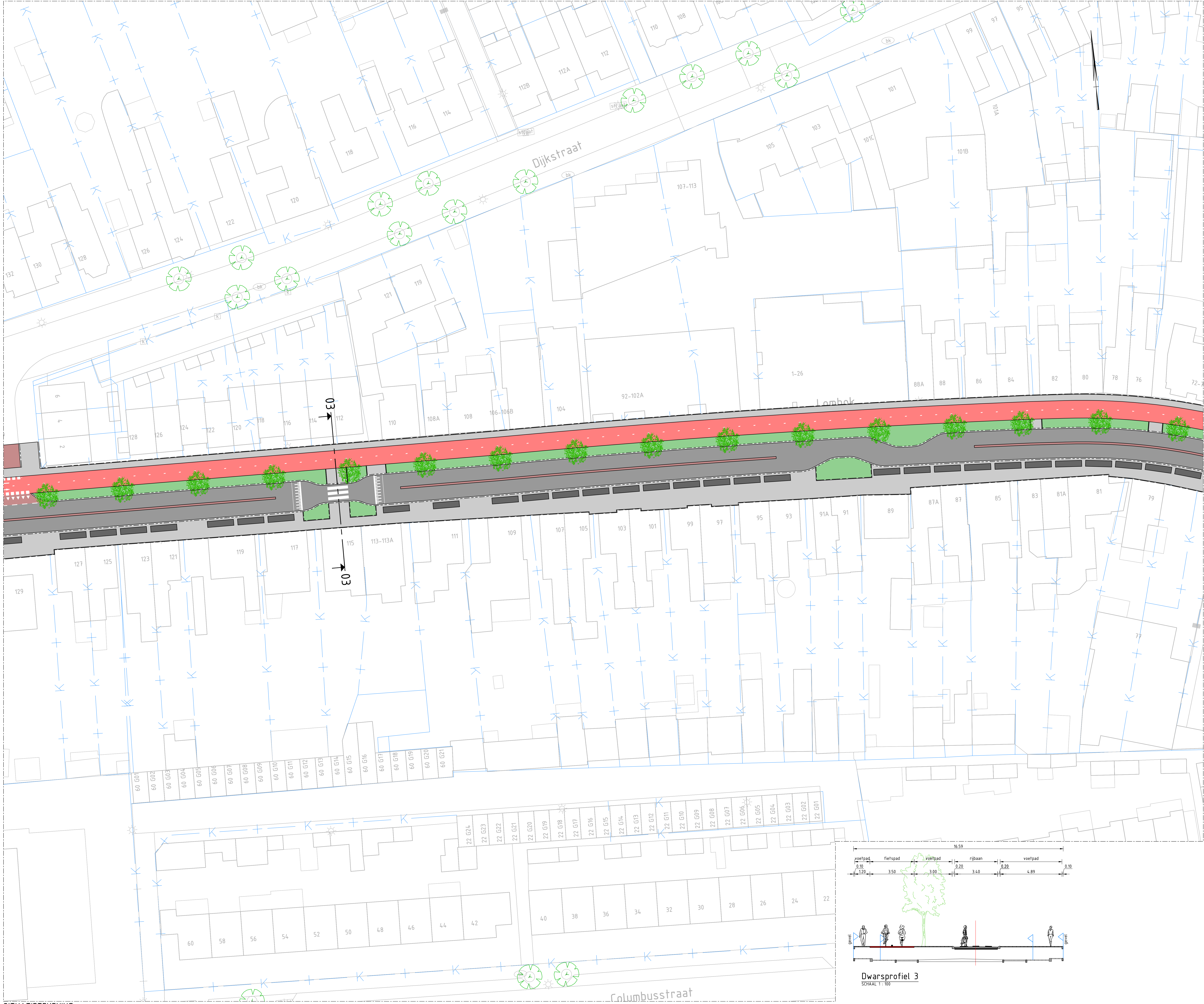
SITUATIETEKENING SCHAAL 1: 250
