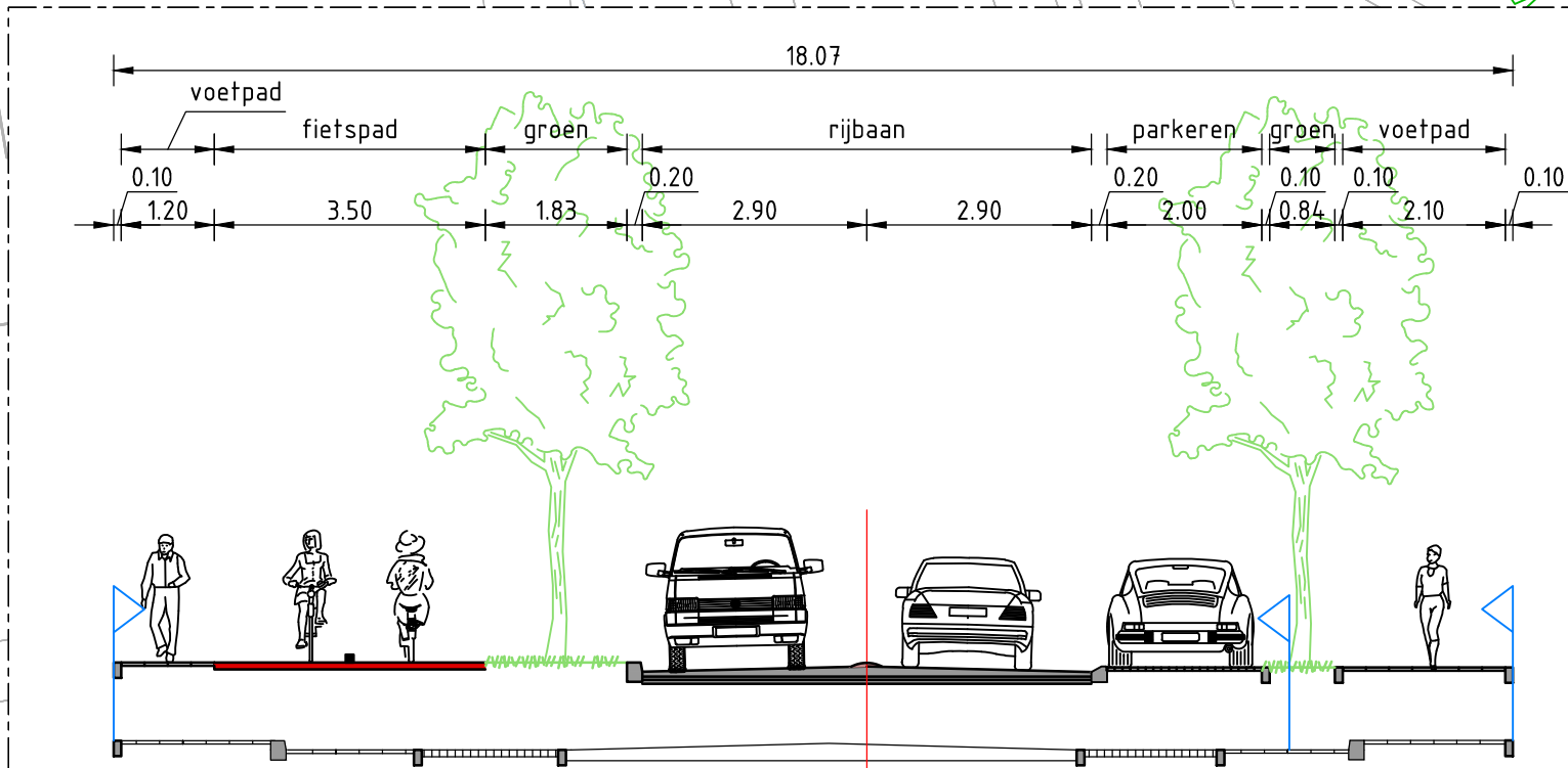
Dwarsprofiel 2 SCHAAAL 1:100
