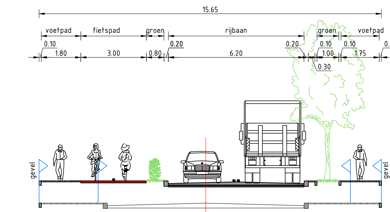
Dwarsprofiel 5 SCHAAL 1:100
