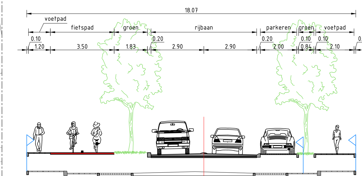
Dwarsprofiel 2 SCHAAF 1:100
