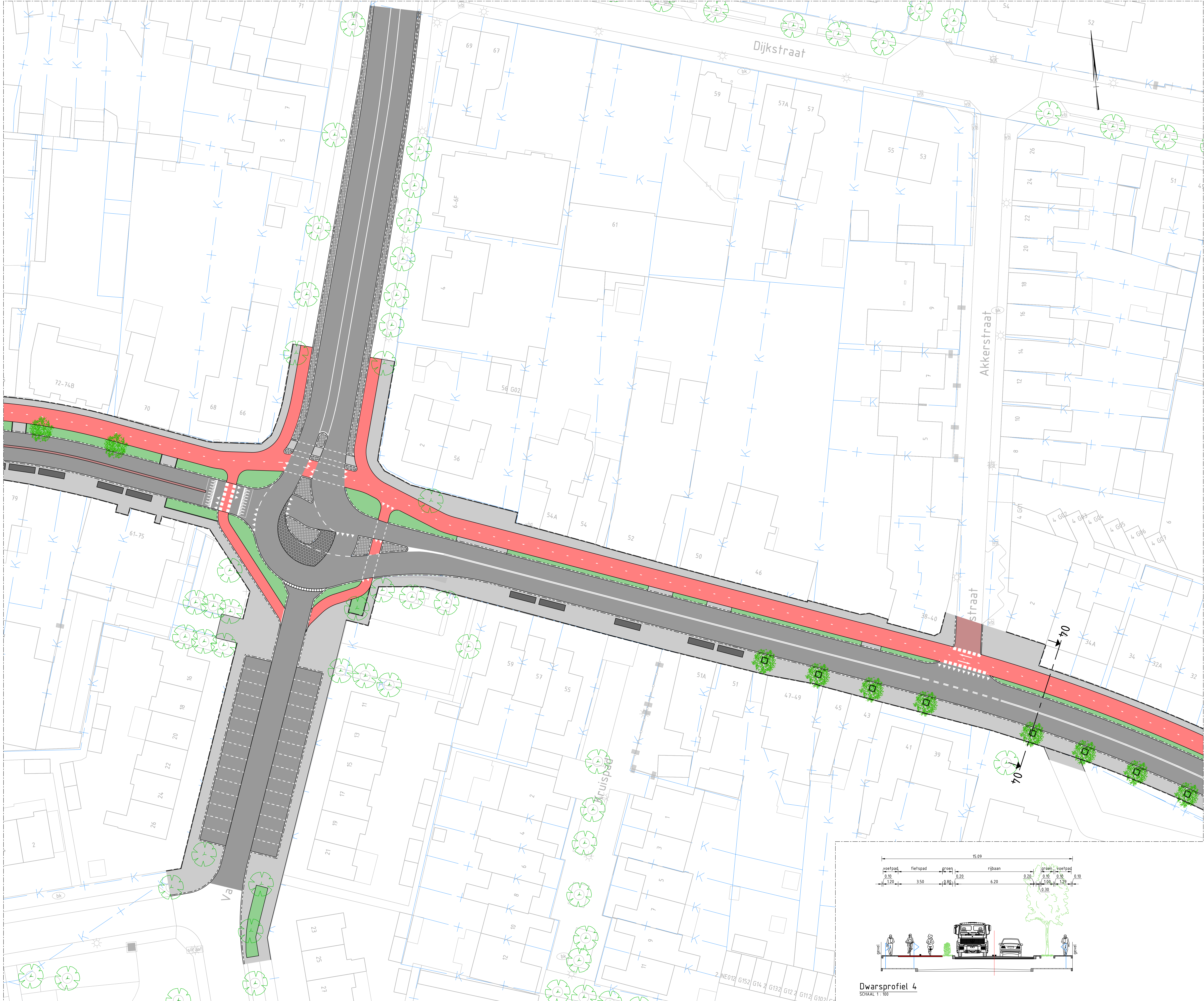
SITUATIETEKENING SCHAALE 1:250
