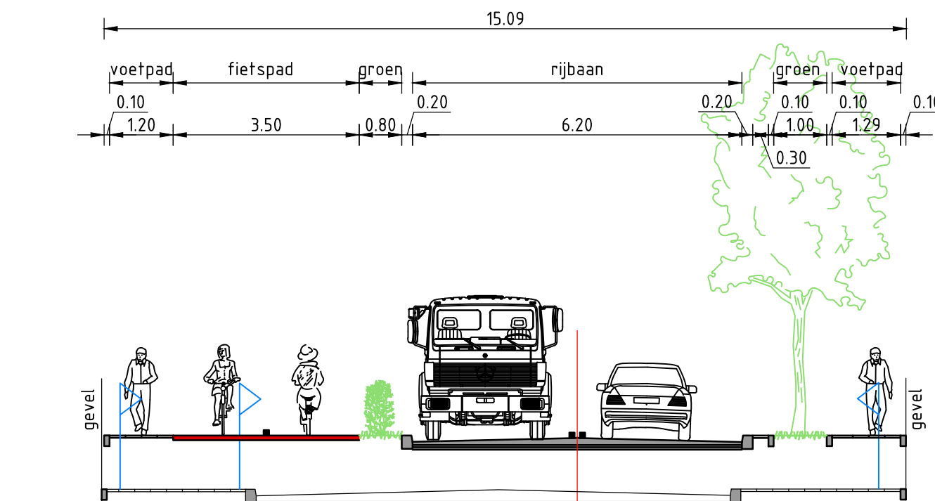
Dwarsprofiel 4 SCHAALE 1:100
