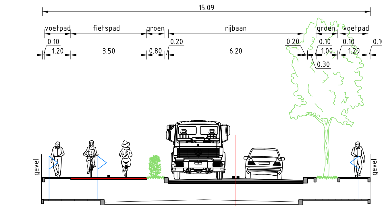
Dwarsprofiel 4 SCHAAL 1:100
