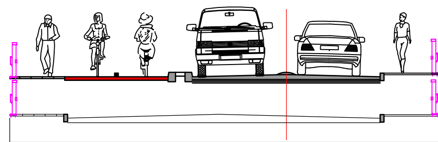
Dwarsprofiel 1 SCHAAL 1:100
