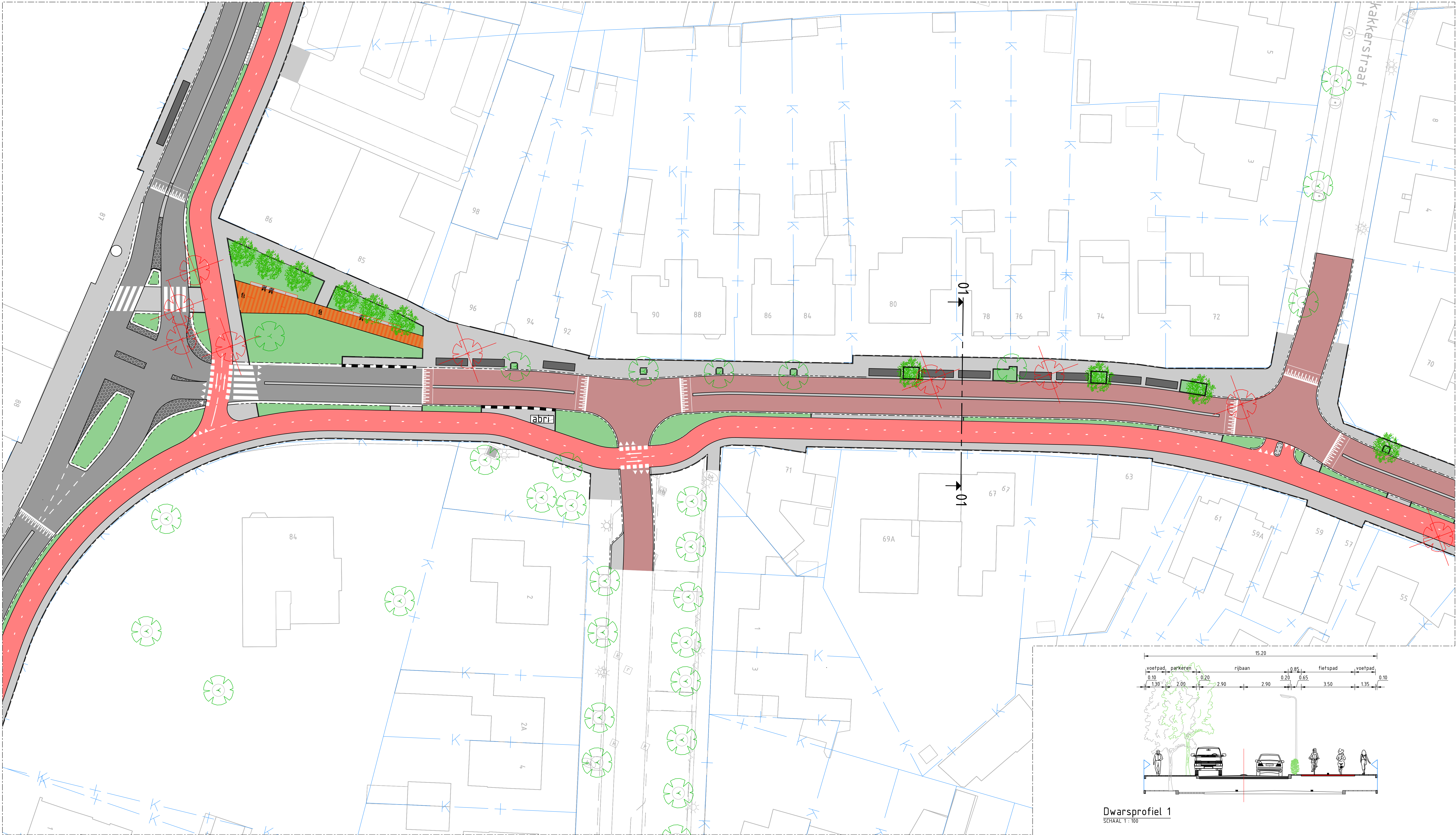
SITUATIE TEKening SCHAAL 1: 250
