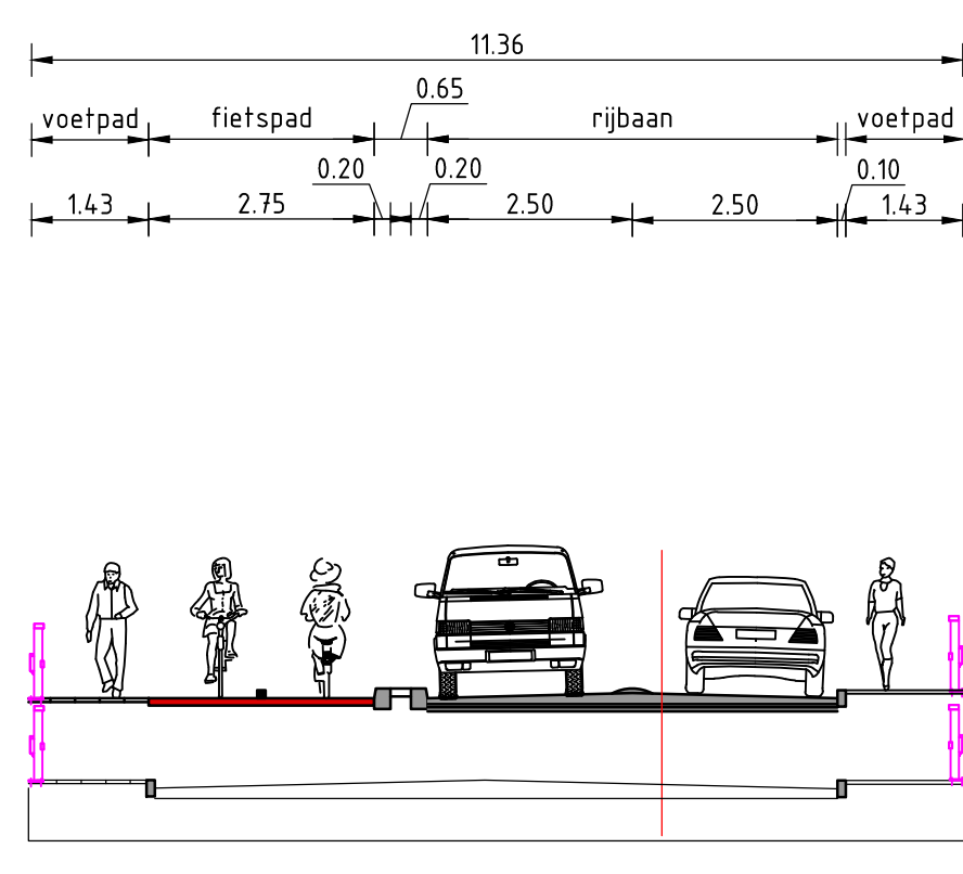
Dwarsprofiel 5 SCHAAL 1:100
