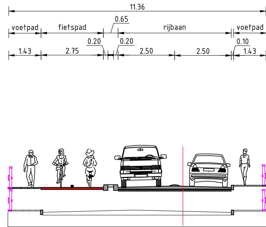
Dwarsprofiel 5 SCHAAL 1:100
