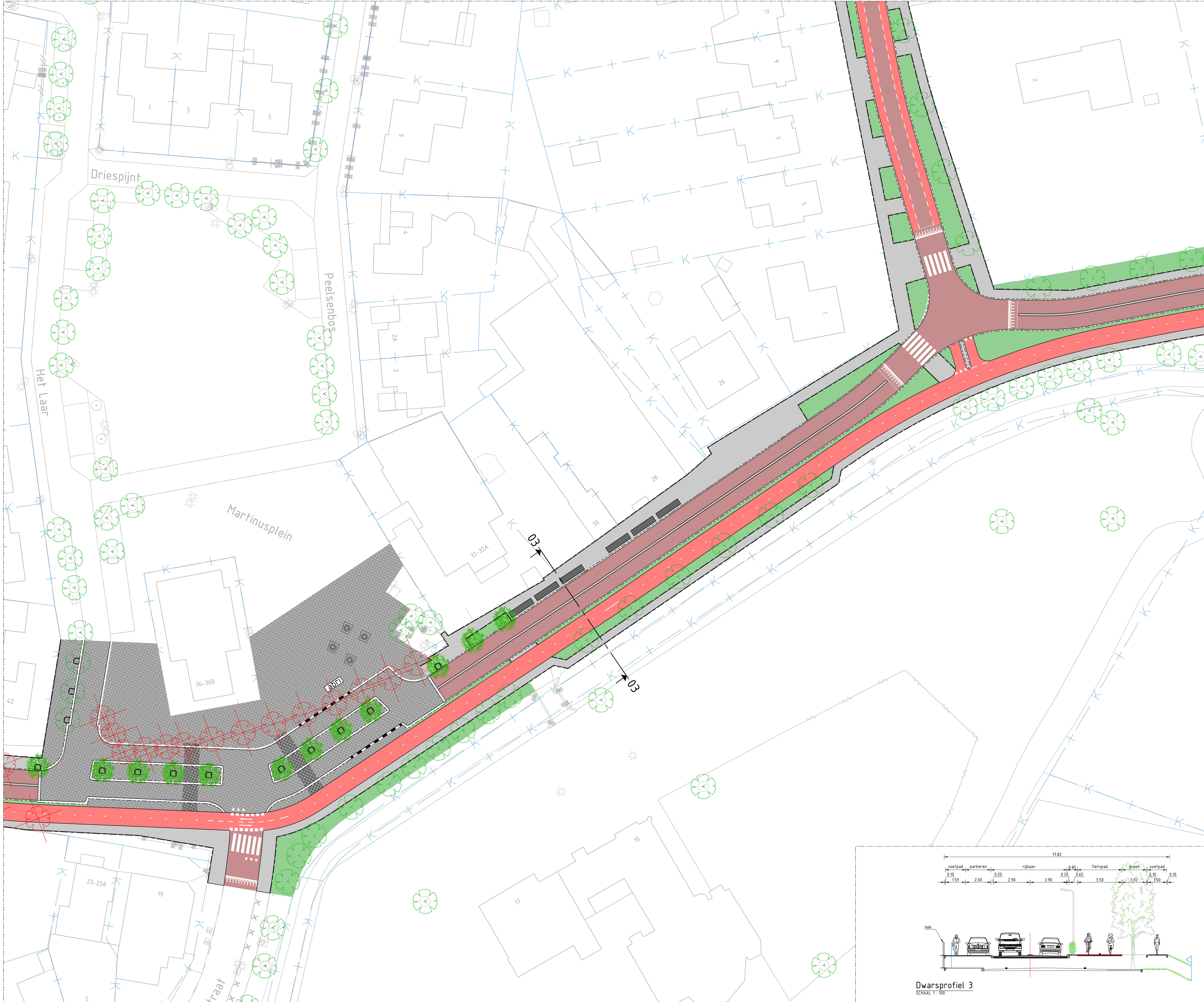
SITUATIE TEKENING SCHAAL 1:250
