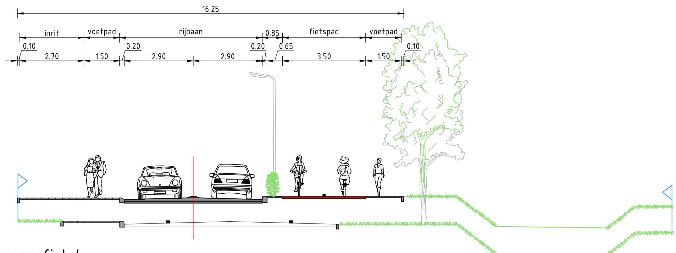
Dwarsprofiel 4 SCHAAL 1:100
