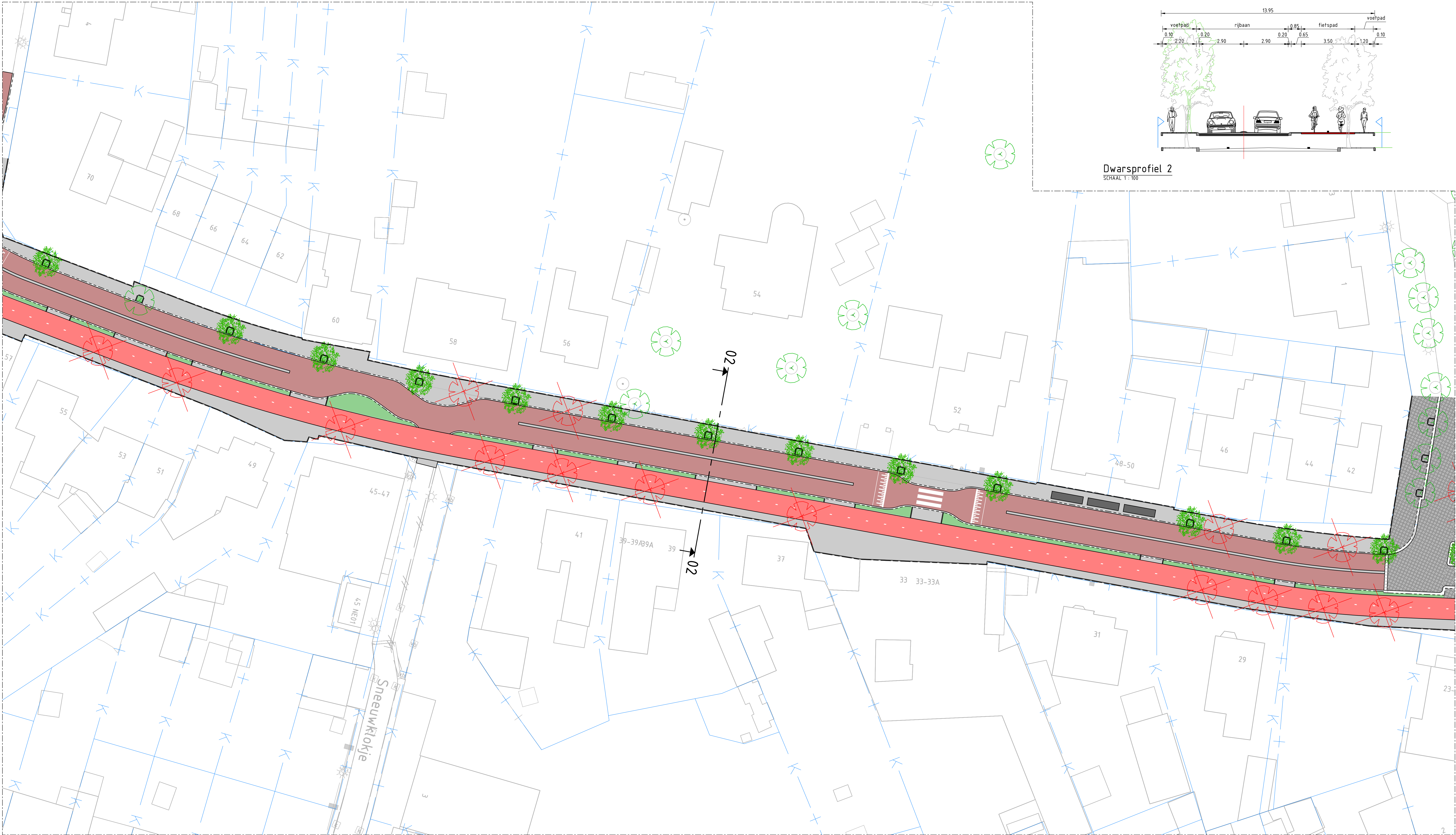
SITUATIEKENING SCHAAL 1 : 250
