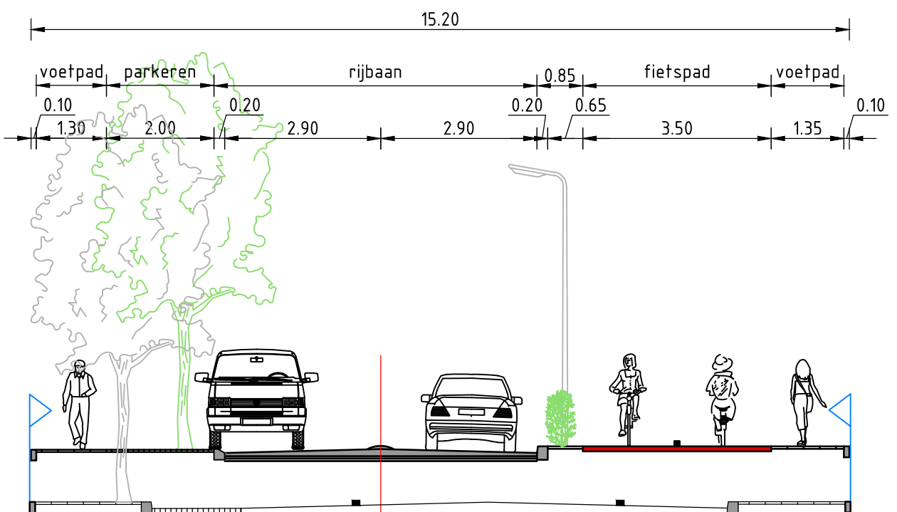
Dwarsprofiel 1 SCHAAL 1: 100
