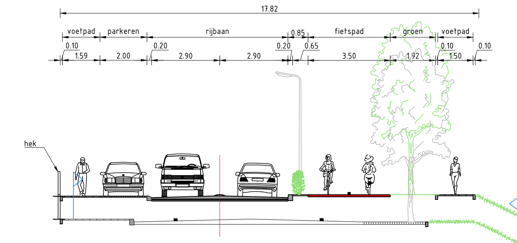
Dwarsprofiel 3 SCHAAL 1:100
