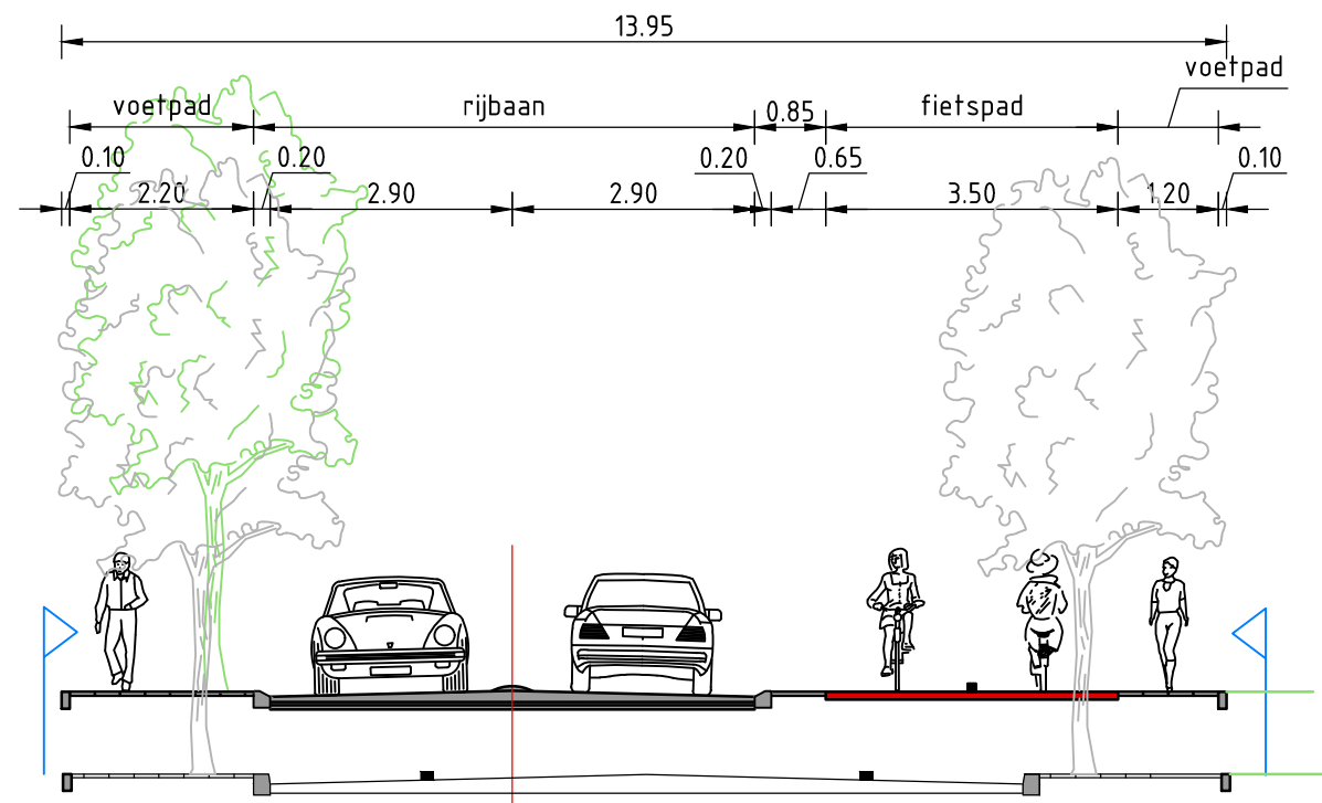
Dwarsprofiel 2 SCHAAL 1 : 100
