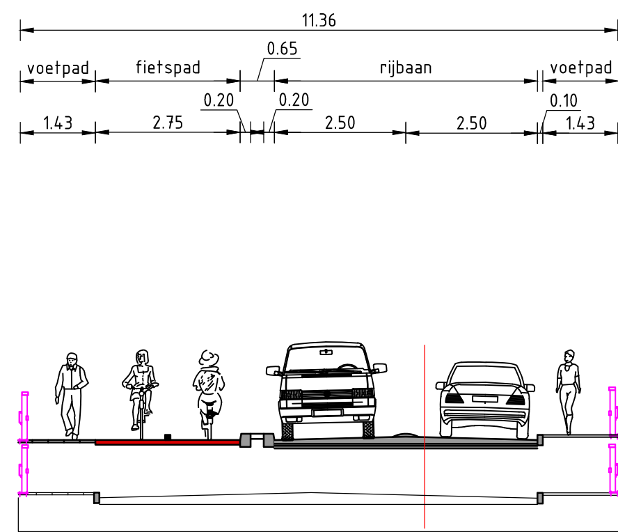
Dwarsprofiel 5 SCHAAL 1:100
