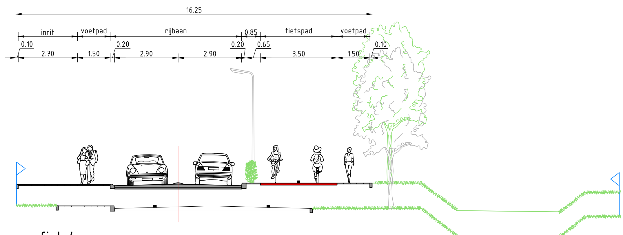
Dwarsprofiel 4 SCHAAL 1:100
